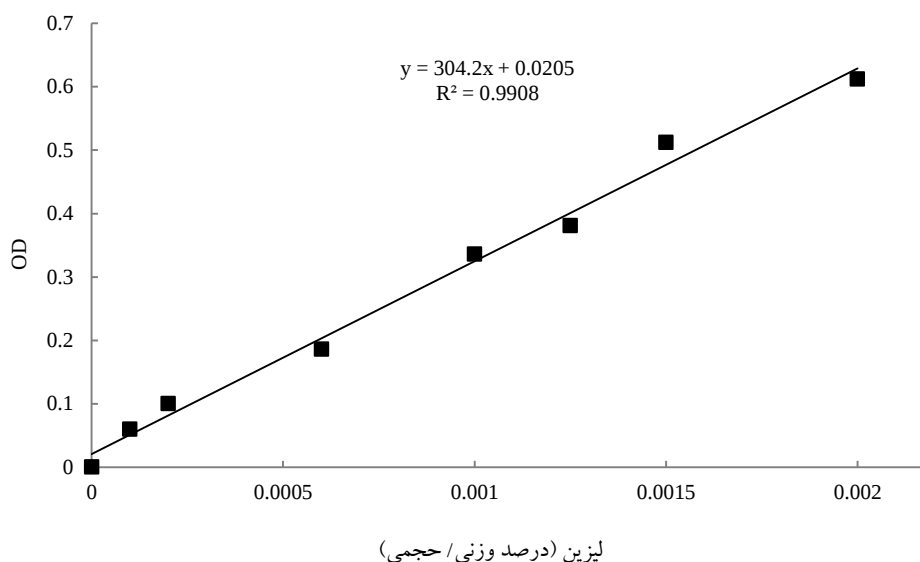
شکل ۱- نمودار استاندارد لیزین. جهت رسم نمودار، غلظت‌های مختلفی از لیزین (درصد‌های مختلف وزنی به حجمی) در آب مقطر تهیه شد سپس با روش چیتارد میزان جذب (OD) نمونه‌ها به دست آمد.
