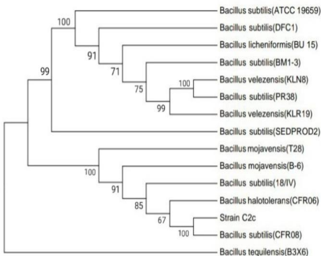
شکل ۶: تجزیه و تحلیل توالی 16S rRNA جدایه C2c به منظور تعیین موقعیت فیلوژنی این باکتری در میان سایر باکتری‌ها در درخت فیلوژنتیکی سویه C2c با استفاده از نرم‌افزار Mega7
