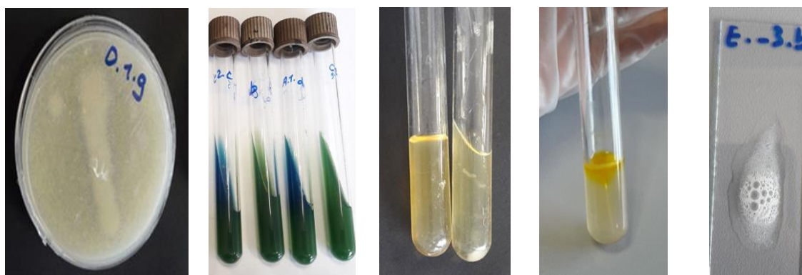
شکل ۲: نتایج تست هیدرولیز قندها از چپ به راست گلوکز، مانیتول، آرابینوز، گزایلو (تغییر رنگ لوله از قرمز نشان‌دهنده مثبت بودن تست است). Figure 2: Results of Sugar Hydrolysis Test (From Left to Right: Glucose, Mannitol, Arabinose, Xylose). A Color Change from Red Indicates a Positive Test.
