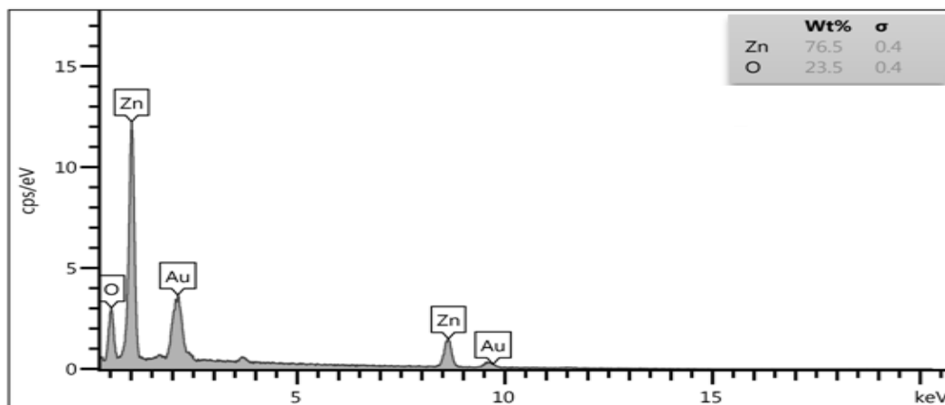
شکل ۵- نمودار EDX نانومیله‌های اکسید روی توسط زانتوموناس کمپستریس
