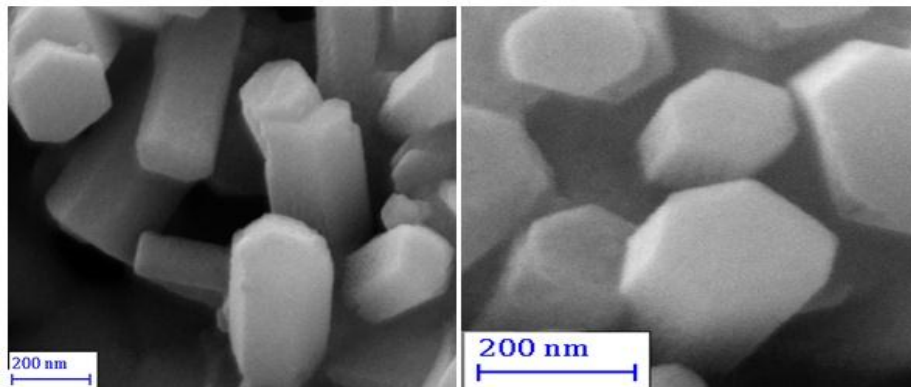
شکل ۴- تصاویر SEM نانومیله‌های اکسید روی به وسیله ی زانتوموناس کمپستریس
