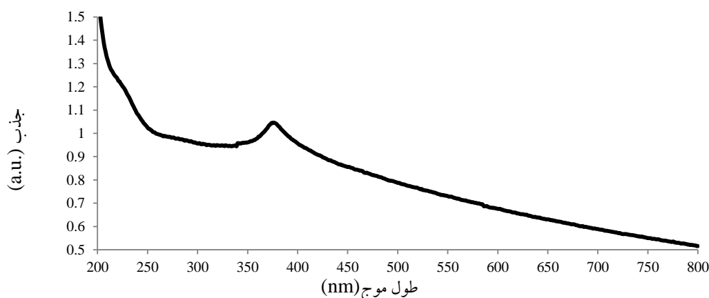
شکل ۶- طیف‌سنجی مرئی- فرابنفش نانومیله‌های اکسید روی توسط زانتوموناس کمپستریس
