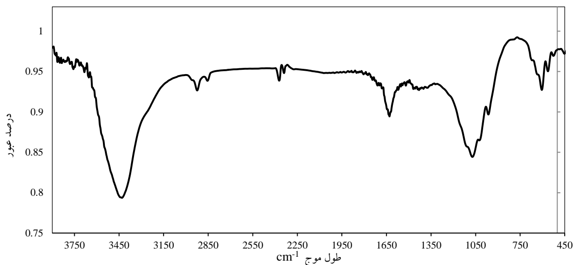
شکل ۲- نمودار FTIR نانومیله‌های اکسید روی سنتز شده توسط زانتوموناس کمپستریس
