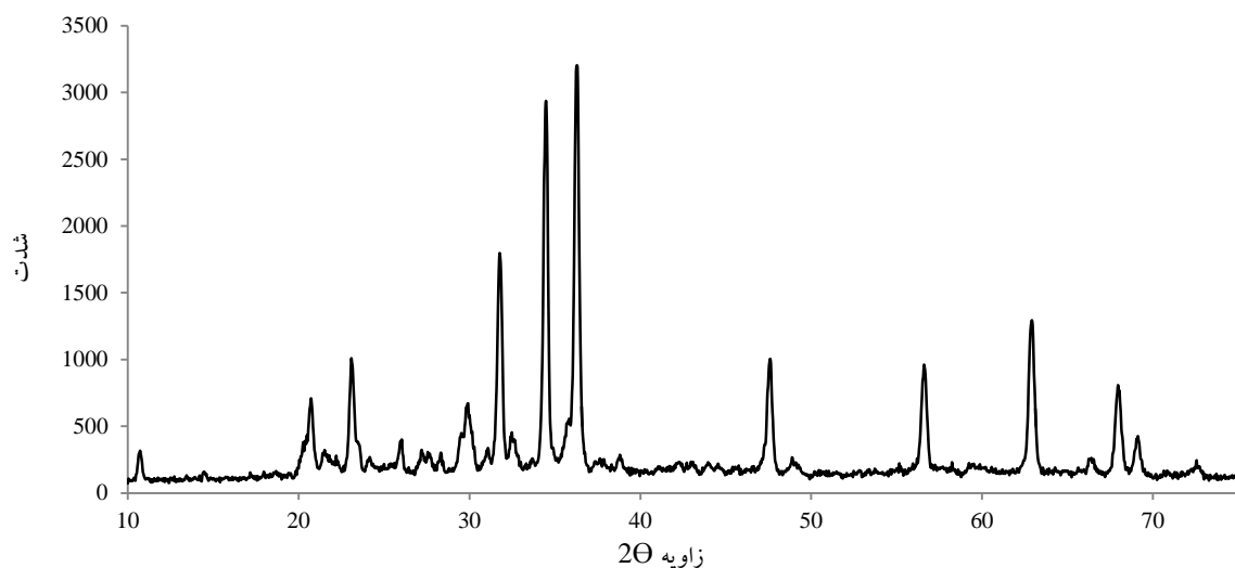
شکل ۳- نمودار XRD نانومیله‌های اکسید روی سنتز شده توسط زانتوموناس کمپستریس
